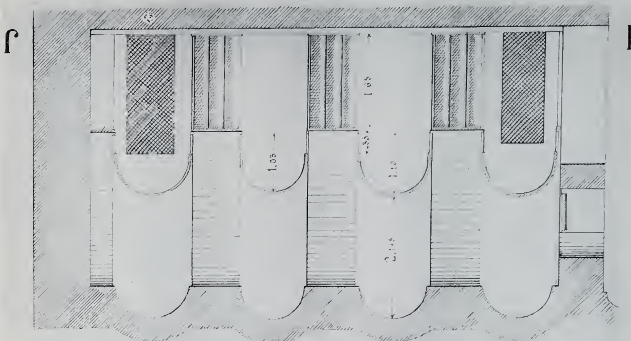
QASR-HARÄNER. - Plan et coupe de la salle 29.
