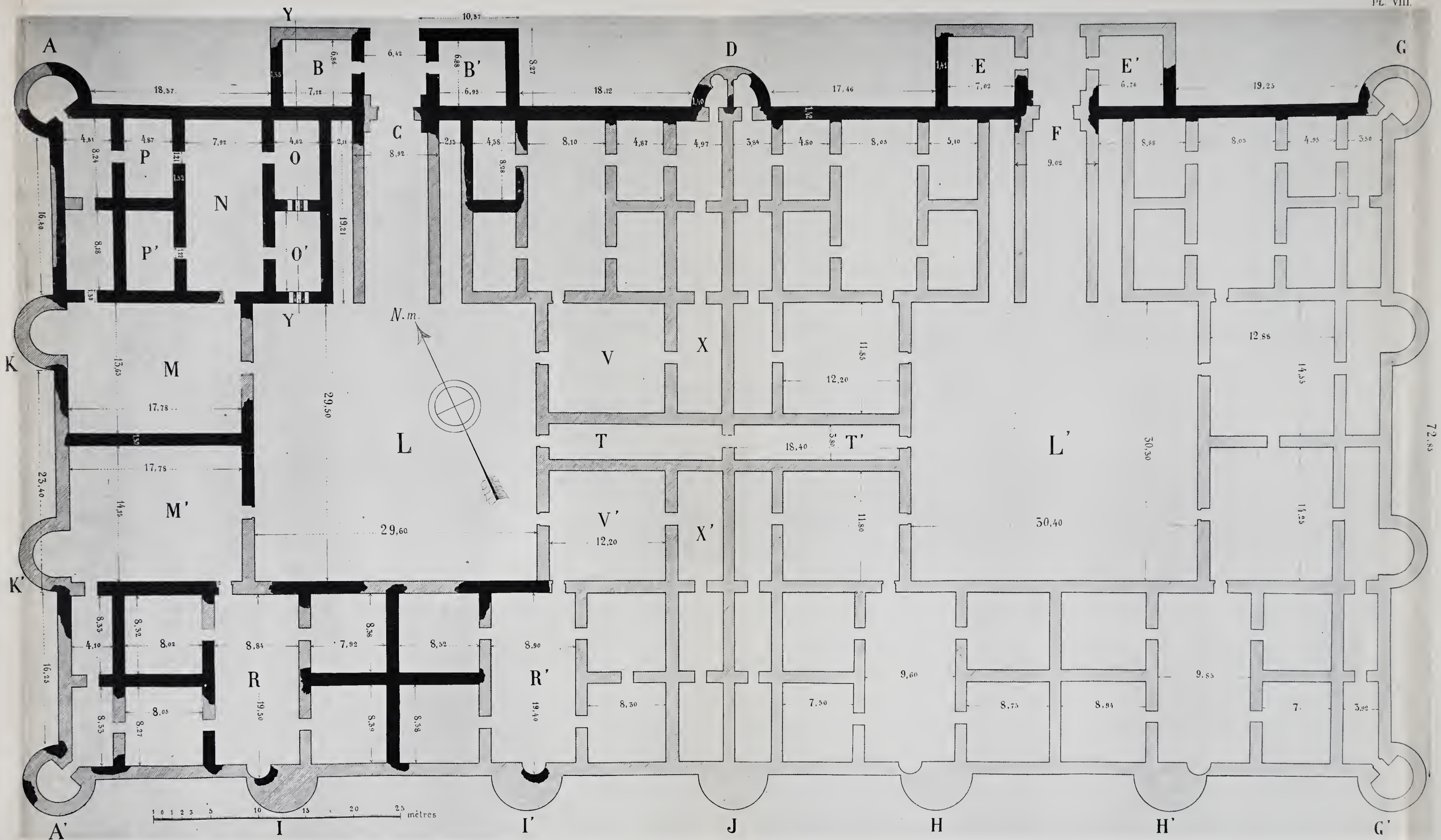
QASR ET-TÔBA. — Plan général des ruines.
