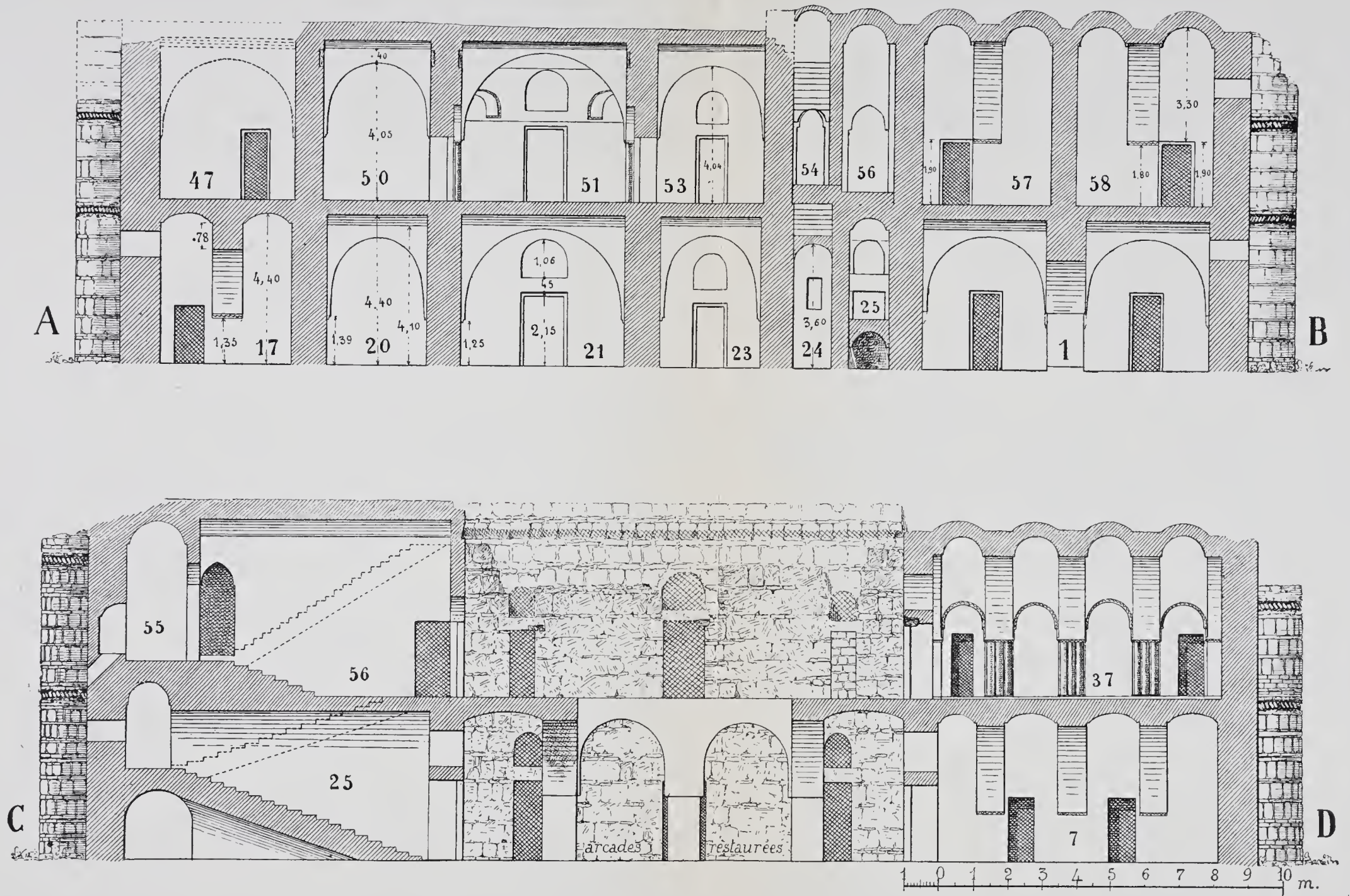
QASR HARANEH. — Coupes sur AB et CD. (Voir les Plans, pl. XXIII et XXIV.)
