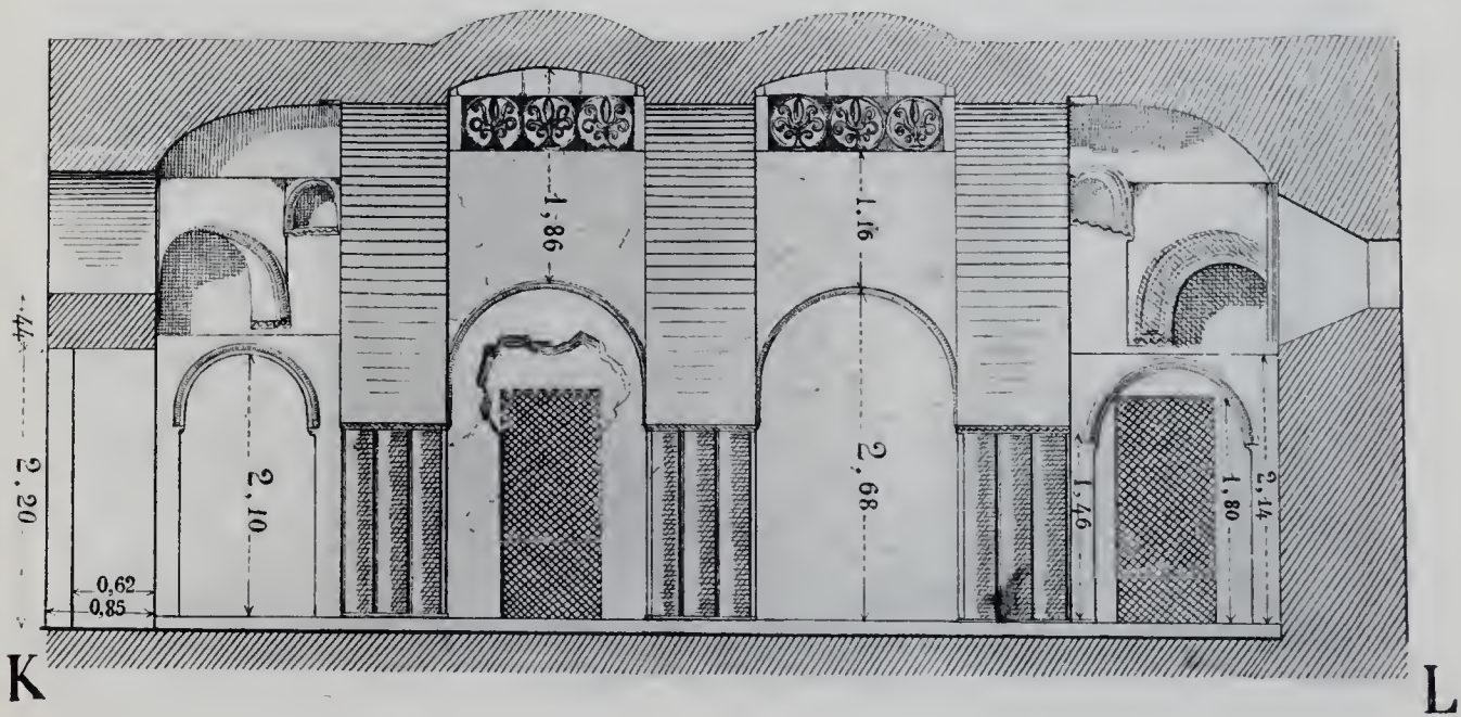
QAŞR-ĪARĀNEH. - Plan et coupe de la salle 51.
